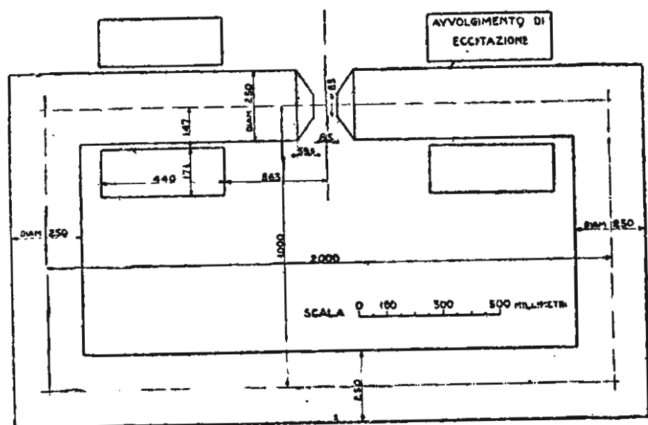
Fig. 4. — Circuito magnetico dei grandi archi.
