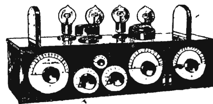
App. ricev. a 4 valvole L. 1500
