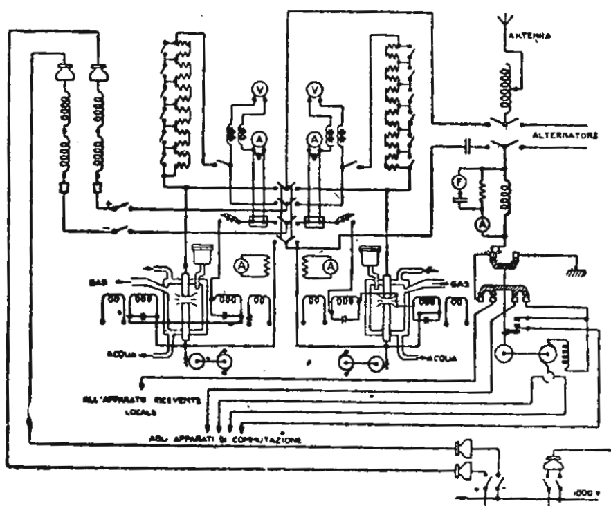
Fig. 6. — Schema di inserzione degli archi.
